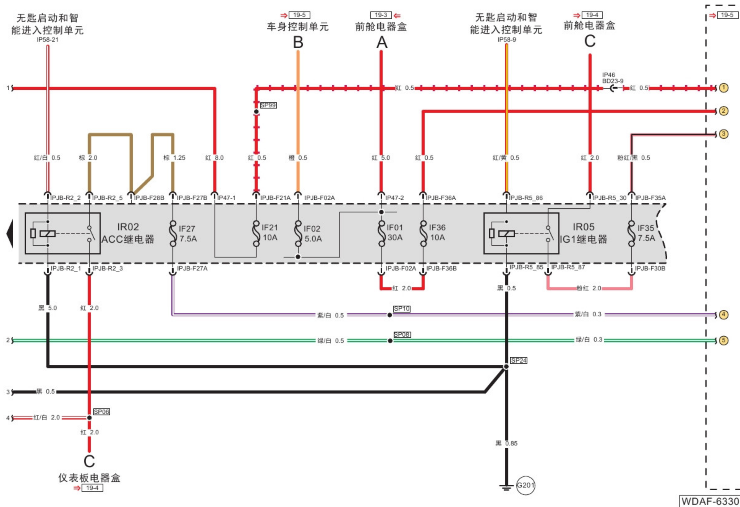
行李箱电路图
